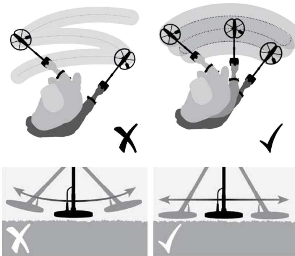
Figure 42 – Balayage de la tête de détection
